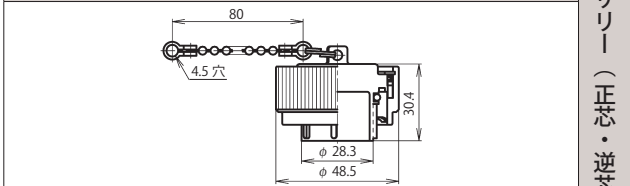
レセプタクルキャップ：BLW-32-RCa
