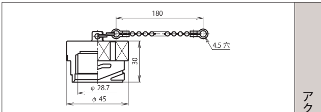
プラグキャップ：BLW-32-PCa
