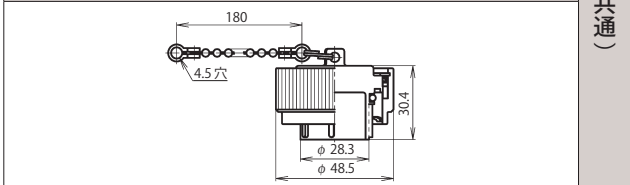
アダプタキャップ：BLW-32-AdCa
