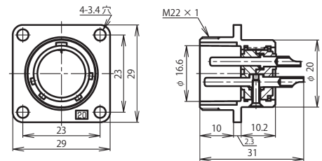
NET-20 ■ -RM
