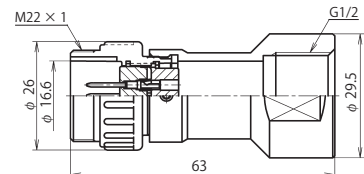
NJW-20 ■ -GAdM1/2 (注)
