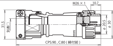
NJW-24 ■ -PMK □
