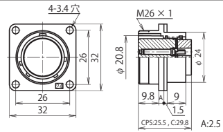
NJW-24 ■ -RF
