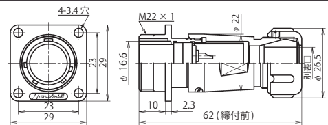
NJW-20 ■ -Ad(F)F □
