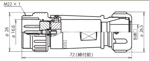
NJW-20 ■ -AdM □
