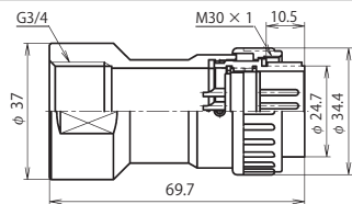
NJW-28 ■ -GPM3/4 (注)
