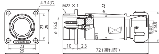
NJW-20 ■ -Ad(F)M □
