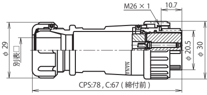
NJW-24 ■ -PF □
