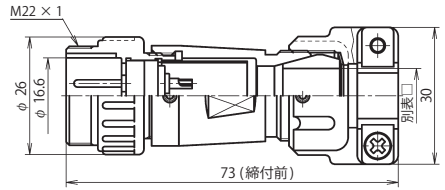
NJW-20 ■ -AdMK □
