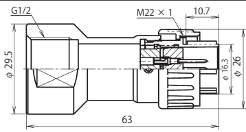
NJW-20 ■ -GPM1/2 (注)
