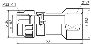
NJW-20 ■ -GAdM1/2 (注)
