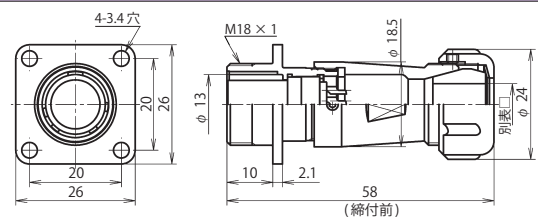
NJW-16 ■ -Ad(F)F □
