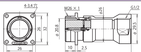
NJW-24 ■ -GAd(F)F1/2 (注)
