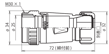
NJW-28 ■ -AdF □
