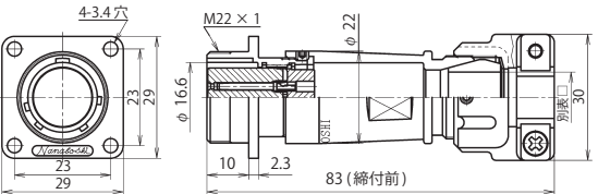
NJW-20 ■ -Ad(F)FK □
