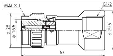
NJW-20 ■ -GAdF1/2 (注)
