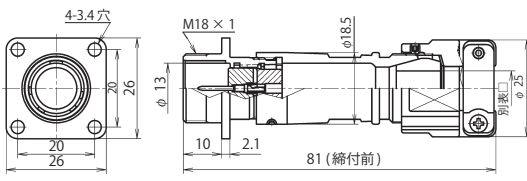
NJW-16 ■ -Ad(F)MK □
