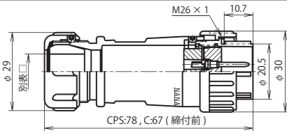
NJW-24 ■ -PM □
