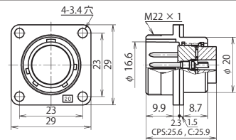
NJW-20 ■ -RM
