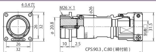
NJW-24 ■ -Ad(F)FK □
