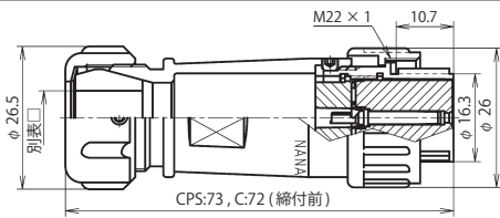
NJW-20 ■ -PF □
