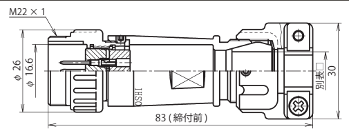
NJW-20 ■ -AdMK □
