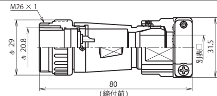
NJW-24 ■ -AdFK □
