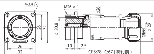
NJW-24 ■ -Ad(F)F □
