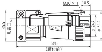
NJW-28 ■ -PMK □
