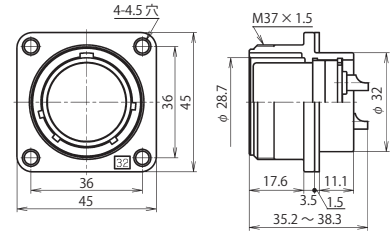
NJW-32 ■ -RF
