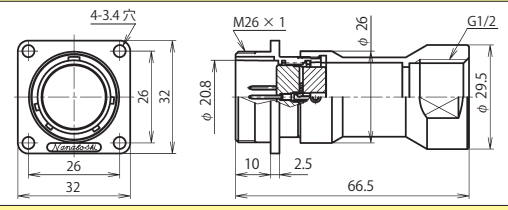
NJW-24 ■ -GAd(F)M1/2 (注)
