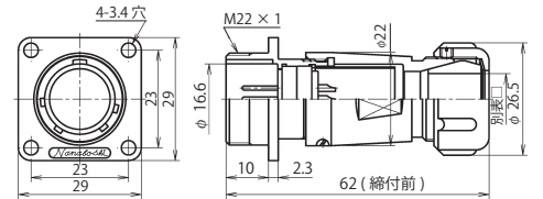
NJW-20 ■ -Ad(F)M □
