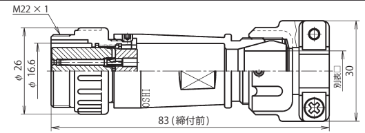
NJW-20 ■ -AdFK □
