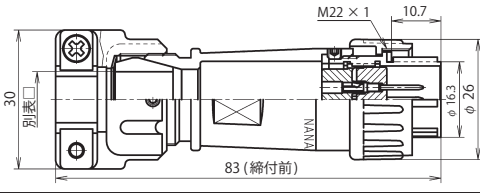
NJW-20 ■ -PMK □
