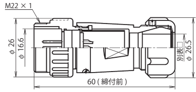
NJW-20 ■ -AdM □
