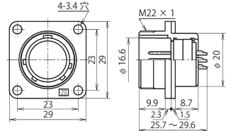
NJW-20 ■ -RM
