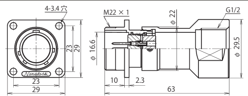
NJW-20 ■ -GAd(F)M1/2 (注)
