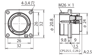
NJW-24 ■ -RM
