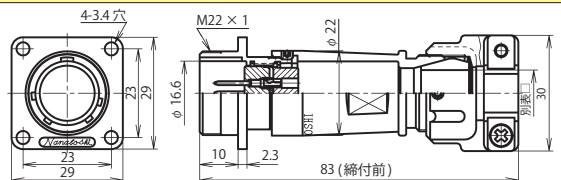
NJW-20 ■ -Ad(F)MK □
