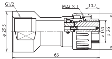
NJW-20 ■ -GPF1/2 (注)
