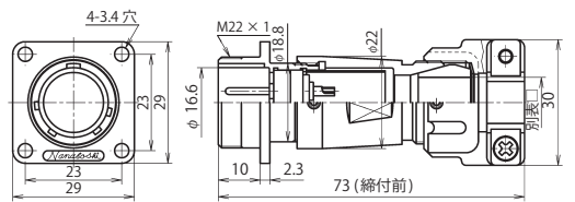
NJW-20 ■ -Ad(F)MK □
