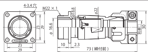
NJW-20 ■ -Ad(F)FK □
