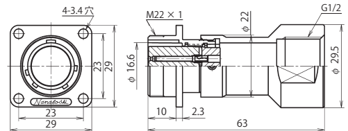
NJW-20 ■ -GAd(F)F1/2 (注)
