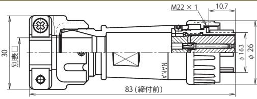
NJW-20 ■ -PFK □
