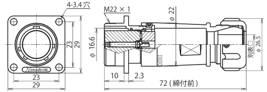
NJW-20 ■ -Ad(F) □
