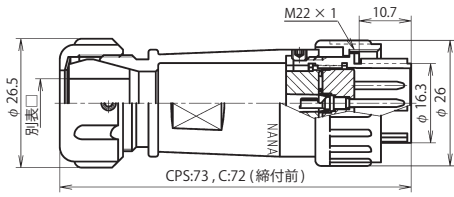
NJW-20 ■ -PM □
